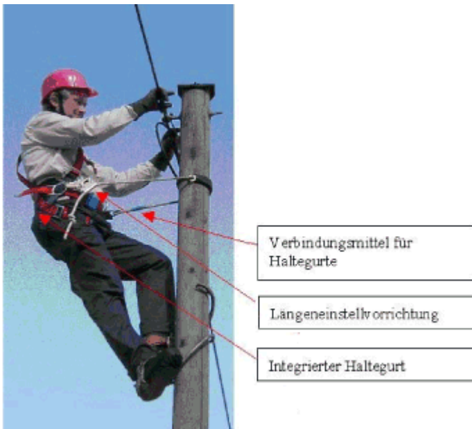
Bild 4: Arbeitsplatzpositionierung an einem Mast durch einen Auffanggurt mit integrierter Haltefunktion
