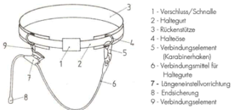
Bild 1: Haltegurt mit Verbindungsmittel für Haltegurte
