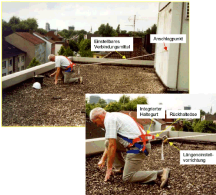
Bild 3: Auffanggurt mit integrierter Rückhaltefunktion und längeneinstellbarem Verbindungsmittel
