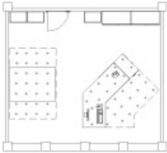
Bild 10: Beispiel für die Verteilung von Messpunkten für eine orientierende Messung. Ermittelt wird die mittlere horizontale Beleuchtungsstärke an zwei Arbeitsbereichen im Büro
