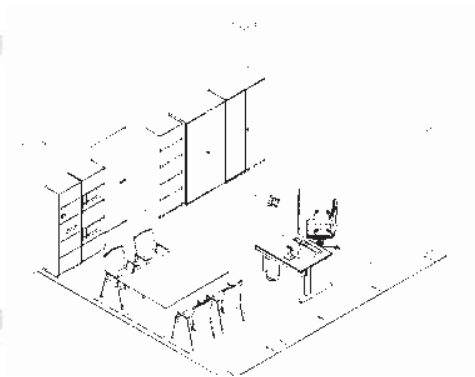
Bild 10: Beispiel für die Verteilung von Messpunkten für eine orientierende Messung. Ermittelt wird die mittlere horizontale Beleuchtungsstärke an zwei Arbeitsbereichen im Büro
