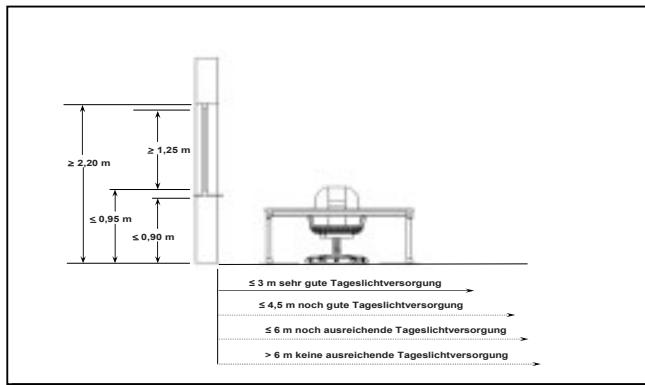
Bild 1: Beispiel für die Tageslichtversorgung in Abhängigkeit von der Raumtiefe (gilt für Räume, in denen die Fensterfront nahezu über die gesamte Raumbreite reicht)
