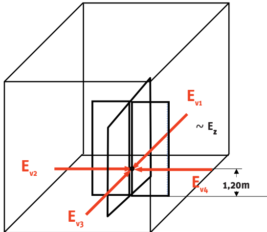
Bild 9: Schematische Darstellung zur Berechnung und Messung der mittleren vertikalen Beleuchtungsstärke in einem Punkt zur näherungsweise Bestimmung der zylindrischen Beleuchtungsstärke
