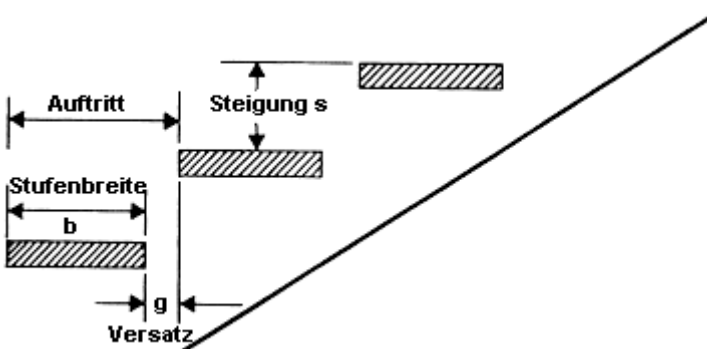
Bild 1c: Treppe mit Versatz
