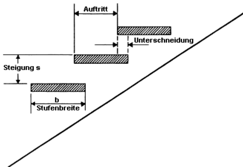
Bild 1b: Treppe mit Unterschneidung
