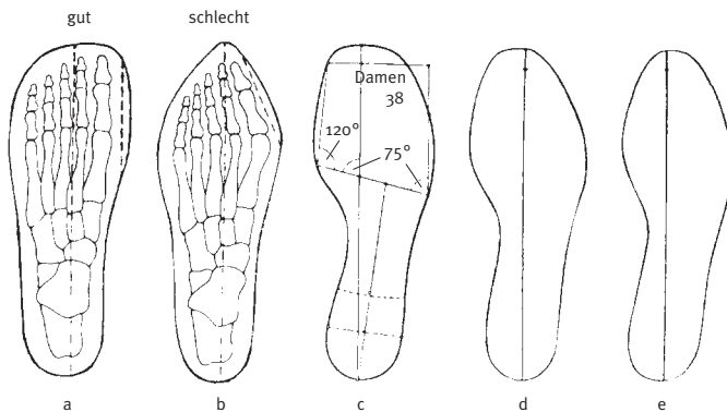
Bild 5: Brandsohlenformen
