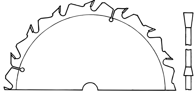
Flachzahn für Längsschnitte
