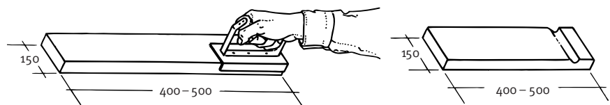
Abb. 30: Schiebehölzer
