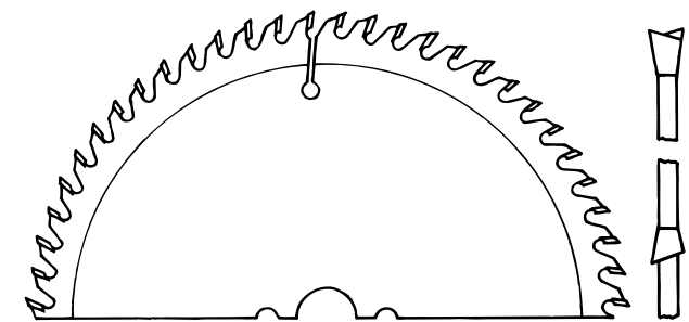
Trapezzahn für Kunststoffe
