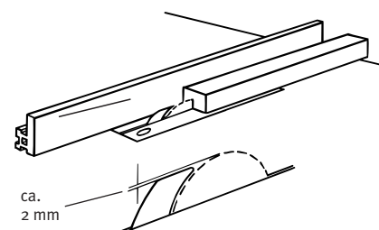
Abb. 26: Verdecktschneiden: Nuten
