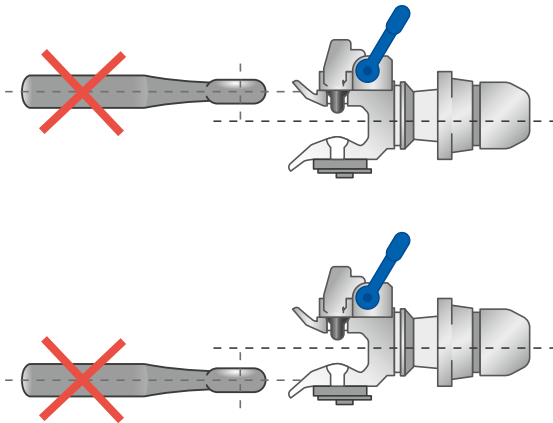
Abb. 13 Zugöse ist zu hoch bzw. zu niedrig eingestellt
