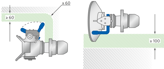
Abb. 3 Mindestmaße für Freiräume in mm zur Betätigung der Bolzenkupplung nach DGUV Vorschrift 70 und 71
