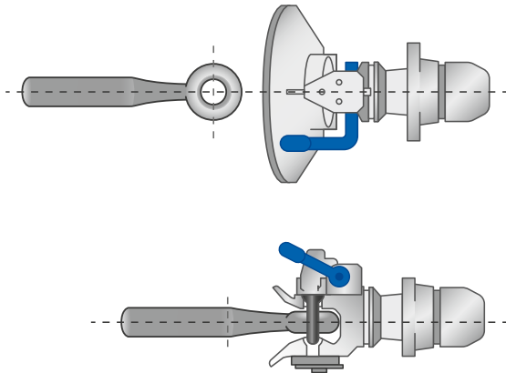
Abb. 15 Zugöse in optimaler Position
