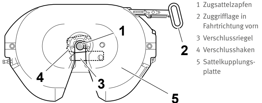
Abb. 8 Bauteile und Funktionsprinzip der Sattelkupplung
