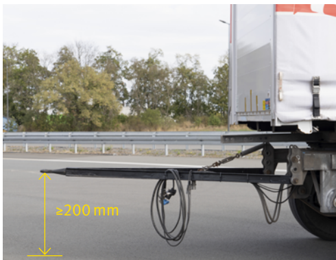
Abb. 4 Mindestbodenfreiheit 200 mm
