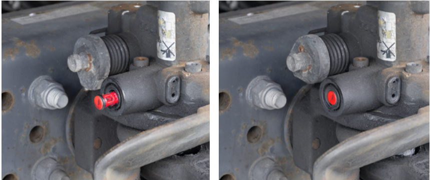
Abb. 2 Kontrollanzeige in geöffneter und geschlossener Stellung der Kupplung
