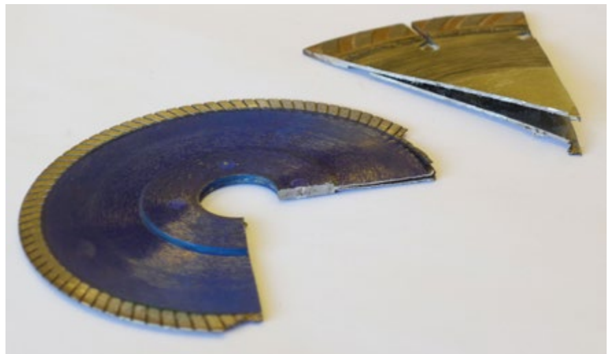
Abb. 3 Aufgeschnittene Diamant-Trennscheiben in Sandwich-Konstruktion
