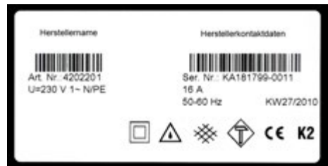
Abb. 2: Geeigneter Leitungsroller und Typschild mit notwendigen Angaben
