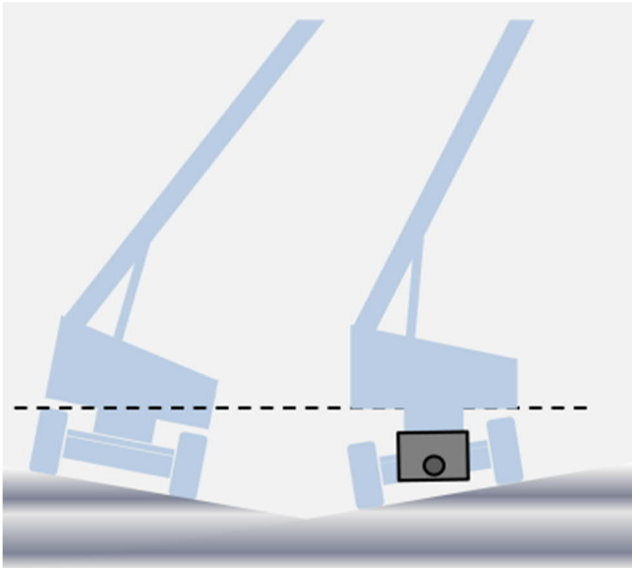
Bild 9: Selbstfahrbühnen ohne und mit Niveaueinstellung
