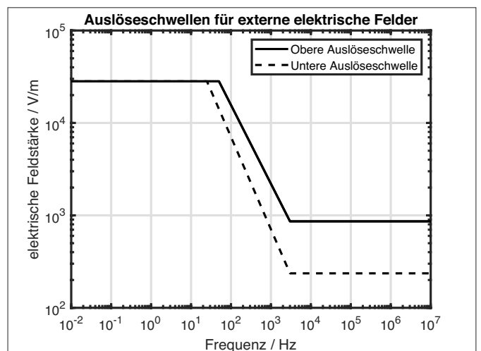
Abbildung 1: Darstellung der Auslöseschwellen für externe elektrische Felder aus Tabelle 7
