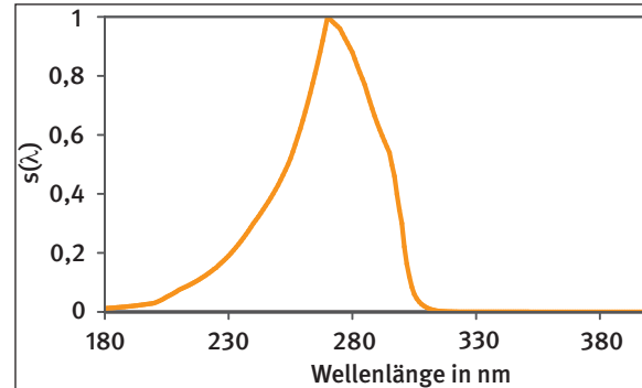
Abbildung 1: Spektrale Wichtungsfunktion S(\lambda)
