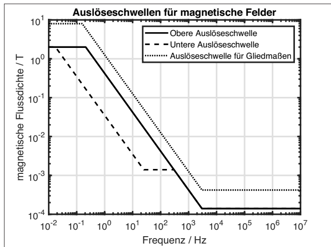
Abbildung 2: Darstellung der Auslöseschwellen für magnetische Felder aus Tabelle 8
