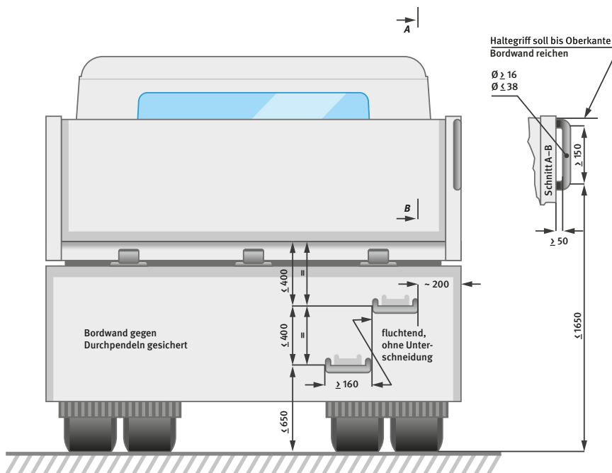
Abb. 3 Klappritt-Aufstiege an einer Bordwand (Maßangaben in mm)
