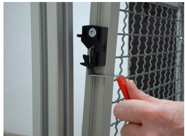
Abbildung 3 – Zertifiziertes Befestigungsmittel für feststehende trennende Schutzeinrichtungen, das nur mit speziellem Werkzeug geöffnet werden kann.
