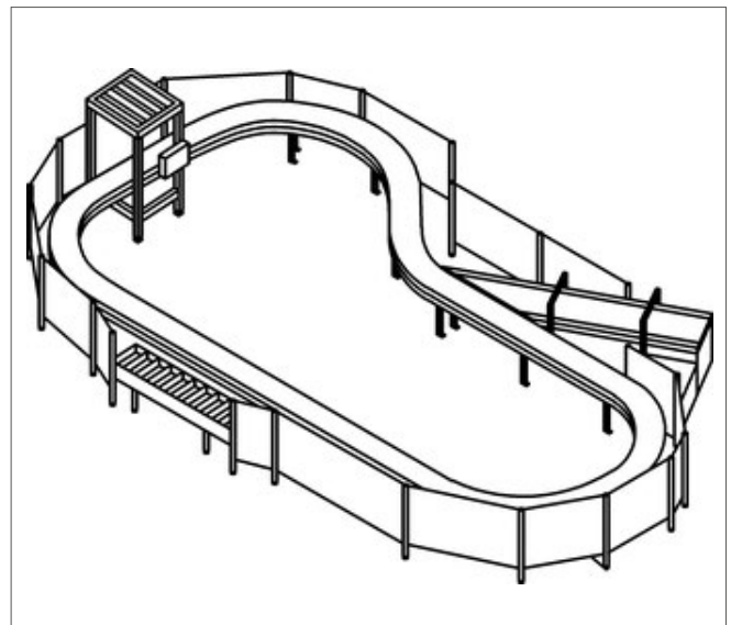
Abb. 9 Loop-Sorter
