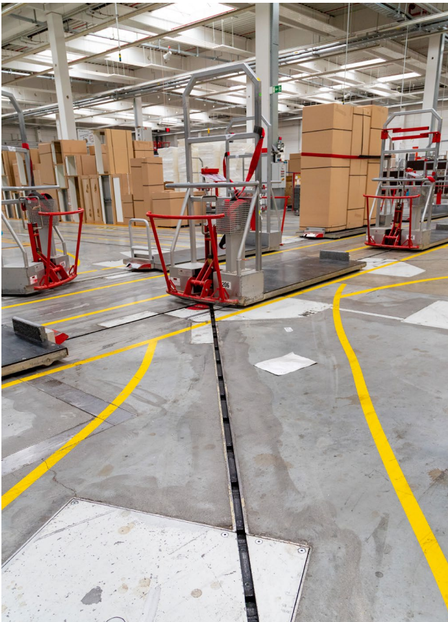
Abb. 15 Unterflurkettenförderer
