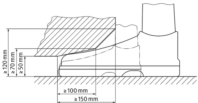
Abb. 37 Fußfreiraum
