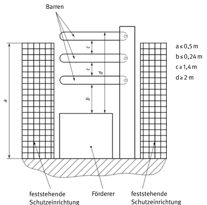
Abb. 29 Zugangssicherung durch Schranke
