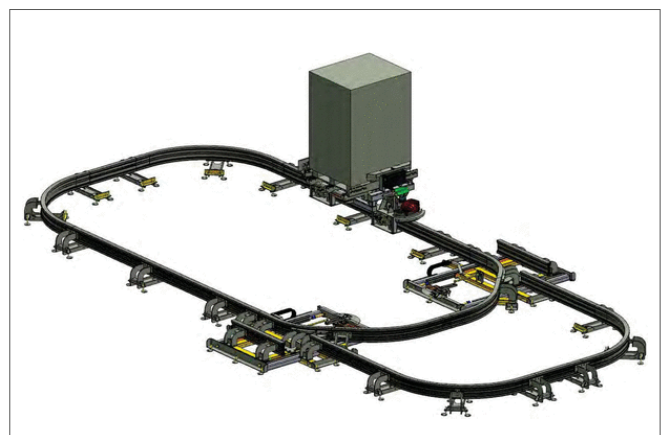
Abb. 10 Einschienen-Bodenförderer
