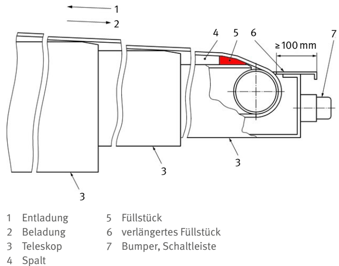
Abb. 36 Kopf des Teleskopförderers mit Schutzeinrichtungen
