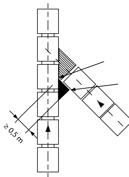
Abb. 55 horizontale Schutzeinrichtung
