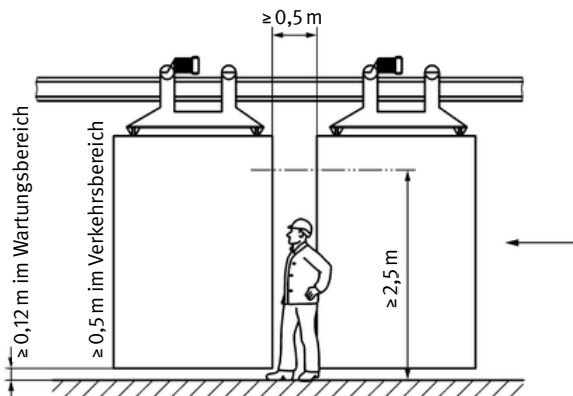
Abb. 40 Abstand in Förderrichtung und zum Boden
