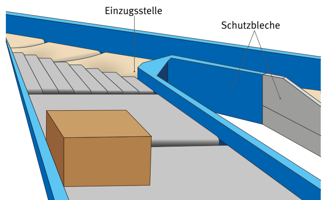
Abb. 54 vertikale Schutzeinrichtung
