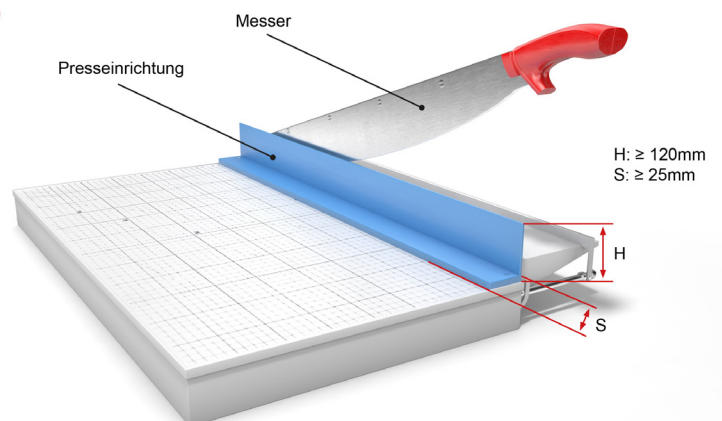
Abb. 8 Presseeinrichtung
