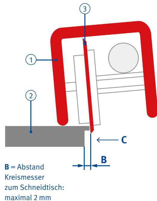
Abb. 14 Messerkopf
