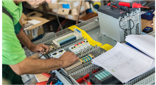
Abb. 21 Verdrahtung eines Schaltschranks
