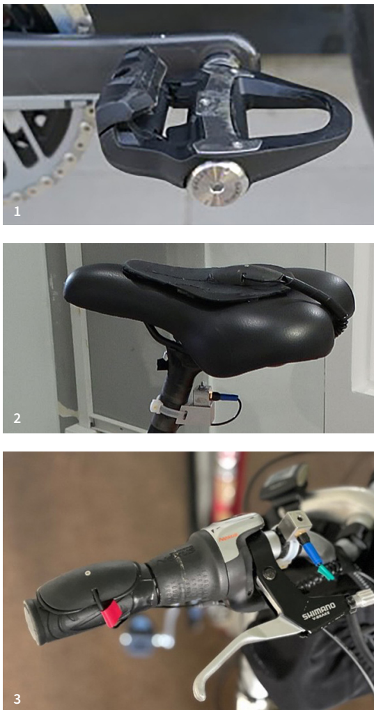
Abbildung 1: Untersuchung der mechanischen und physikalischen Expositionen; 1: Garmin Rally RS200 Powermeter, 2: Beschleunigungsaufnehmer auf dem Sattel und Sattelstütze, 3: Beschleunigungsaufnehmer auf dem Lenkergriff und Lenkerstange
