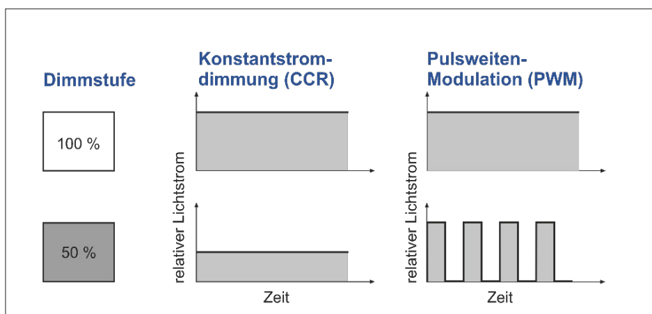
Abbildung 1: Bei der Konstantstrom-Reduktion wird die Helligkeit gleichmäßig reduziert (Mitte). Bei der Pulsweitenmodulation (rechts) wird mit der An-/Aus-Funktionsweise (Hell/Dunkel) gedimmt.
