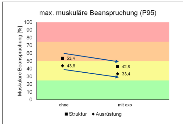
Abbildung 4: Effekt des Exoskeletts auf die muskuläre Schulterbeanspruchung. Einstufung der Montagevorgänge in der Strukturmontage als schwer und in der Ausrüstungsmontage als mittelschwer.
