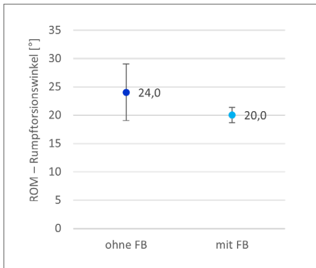
Abbildung 5: ROM-Mittelwert des Rumpftorsionswinkels ( \pm SD) im Transferintervall ohne 24,0 \pm 5,0^\circ (n = 575 Gepäckstücke) und mit FB 20,0 \pm 1,4^\circ (n = 653)
