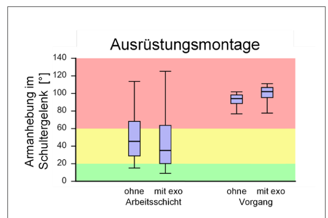
Abbildung 3: Die Analyse der Armhebung im Schultergelenk zeigt keine relevanten Veränderungen, weder in der Verteilung der Armhaltungen über die gesamte Arbeitsschicht noch bei einzelnen Montagevorgängen. Die Montagearbeiten finden überwiegend in kritischen Winkelbereichen des Schultergelenks statt.
