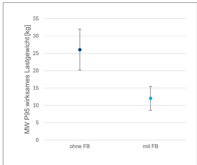
Abbildung 6: P95-Mittelwert ( \pm SD) des wirkenden Lastgewichts im Transferintervall ohne 26,1 \pm 5,9 kg (n = 575 Gepäckstücke) und mit FB 12,0 \pm 3,4 kg (n = 653)
