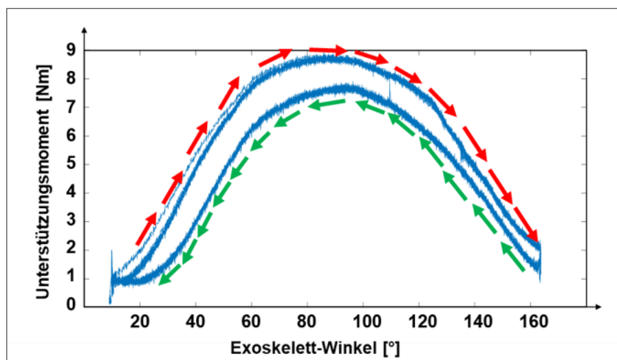
Abbildung 1: Kennlinie des untersuchten Exosketts bei maximaler Unterstützungseinstellung. Dargestellt ist das winkelabhängige Unterstützungsmoment über den Bewegungsbereich des Exosketts. Die roten Pfeile kennzeichnen die Phase der Oberarmabsenkung, während die grünen Pfeile die Oberarmhebung markieren. In der Hebe-Phase treten geringere Unterstützungsmomente auf als in der Absenkungsphase, was eine Hysterese im Systemverhalten zeigt (Energieverlust).
