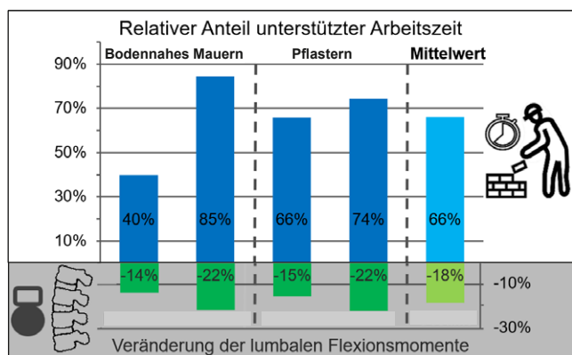
Abbildung 4: Zeitlicher Unterstützungsanteil und relative Entlastung durch Einsatz eines Exoskeletts bei bestimmten Tätigkeiten in der Baubranche
