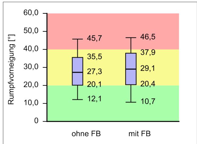
Abbildung 4: Verteilung der Rumpfvorneigung bei der Entladung von n = 43 Frachtcontainern ohne FB und n = 50 mit FB. Hier ist die Vorneigung mit und ohne FB auf ähnlichem Niveau und ragt in den nicht akzeptablen Bereich.
