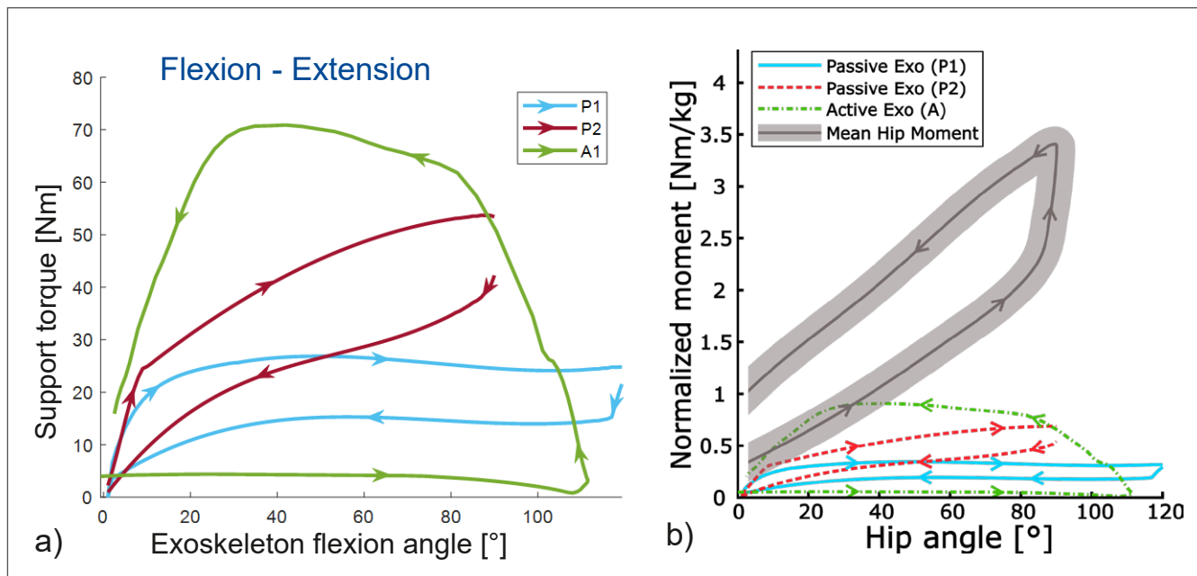
Abbildung 3: a): Kennlinien verschiedener Exoskelette (P1, P2: passiv; A: aktiv) (nach [5]) b): Hüftgelenkmoment beim Anheben einer Last (20 kg) im Vergleich zu den Exoskelett-Kennlinien
