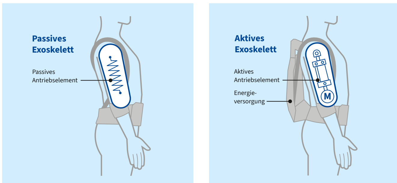
Abbildung 1: Unterscheidung von Exoskeletten nach dem Antriebsprinzip (© DGUV – KonzeptQuartier GmbH)
