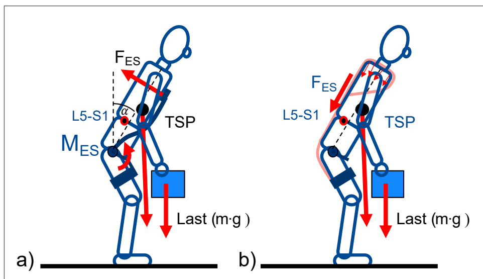
Abbildung 1: Biomechanisches Mehrkörpermodell zur Bestimmung des lumbalen Gelenkmoments um L5/S1 (Last = Gewichtskraft der Last, TSP = Gewichtskraft des Rumpfes einschließlich der des Kopfes, \alpha = Beugewinkel des Exoskeletts, MES = Drehmoment des Exoskeletts, FES = Rückstellkraft des Exoskeletts mit dem Wirkprinzip eines a) starrgliedrigen Exoskeletts und dem eines b) Soft-Exoskeletts. Die im Modell berücksichtigten Trägheitseffekte sind nicht in der Abbildung dargestellt.
