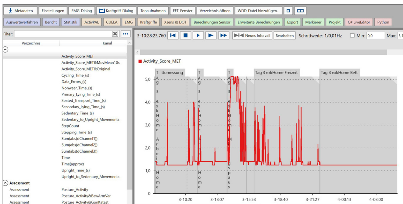
Abbildung 1: Markierung der Intervalle einer Messung mit der CUELA-Software
