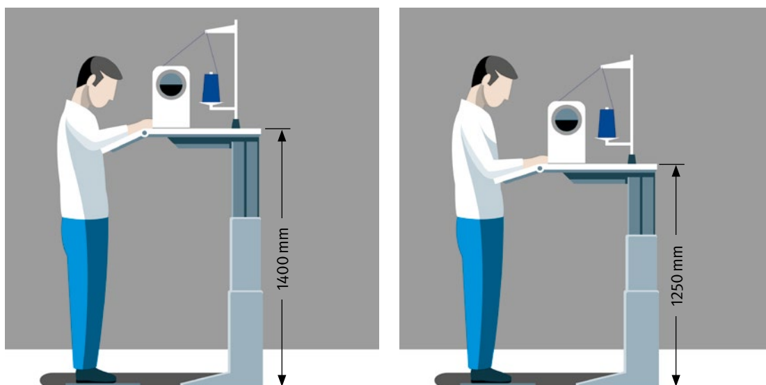
a) bei sehr hohen Genauigkeitsanforderungen (Sehabstand < 300 mm) → Tischhöhe 1400 mm
