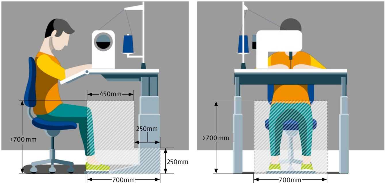
Abb. 6 Mindestmaße für Fuß- und Beinraum beim Sitznäh-arbeitsplatz (* Bezugsebene für die Maßangaben ist die Tischvorderkante)
