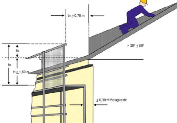
Abb. 7.2.2: Dachfanggerüst gemäß Abs. 4.3.4 Regel „Dacharbeiten“ (BGR 203)
