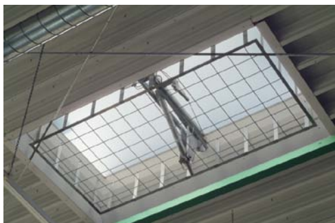
Abb. 7.3.3: Beispiel einer bauseitigen Absturzsicherung an Lichtkuppeln. Im Bereich der Lichtkuppel kann auf temporäre Maßnahmen gegen Absturz auf der Dachfläche verzichtet werden.
