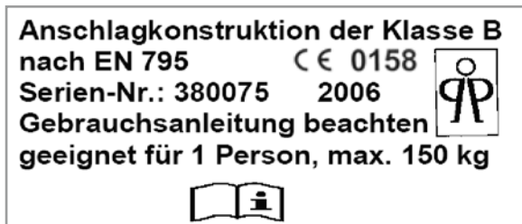
Abb. 5.3.2: Beispiel für die Kennzeichnung einer Anschlagkonstruktion der Klasse B, u.a. mit Hinweis zum Hersteller und zur Beachtung der Gebrauchsanleitung
