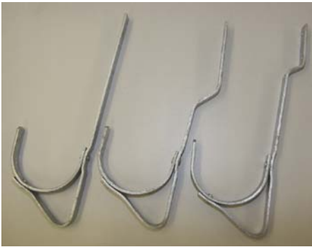
Abb. 5.3.3: Sicherheitsdachhaken nach DIN EN 517 in verschiedener Ausführung für unterschiedliche Einbausituationen.
