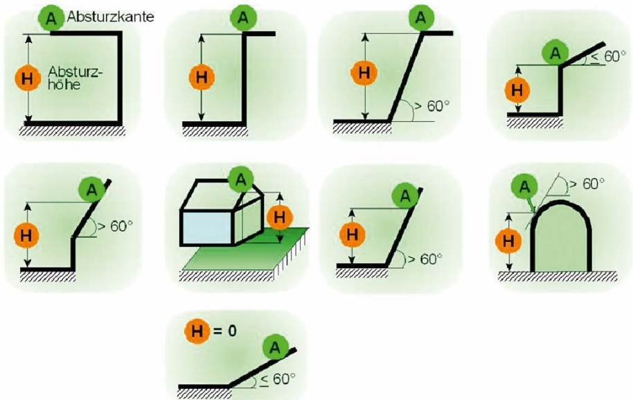
Abb. 7: Absturzhöhen können in Abhängigkeit der Lage des jeweiligen Arbeitsplatzes, der Absturzkante sowie der Auftreffstelle differieren (siehe auch Unfallverhütungsvorschrift „Bauarbeiten“ (BGV/GUV-V C22)).
