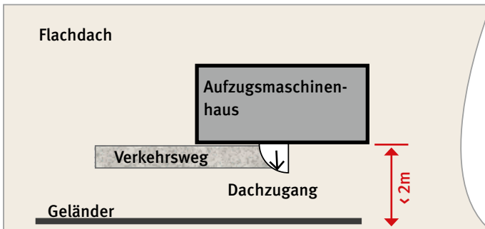
Abb. 5.2.1: Im Beispiel grenzt der Dachzugang unmittelbar an einen Dachbereich mit Absturzgefahr (Abstand des Verkehrsweges zur Dachkante < 2 m). Hier ist als Schutz gegen Absturz z.B. ein Geländer erforderlich.
